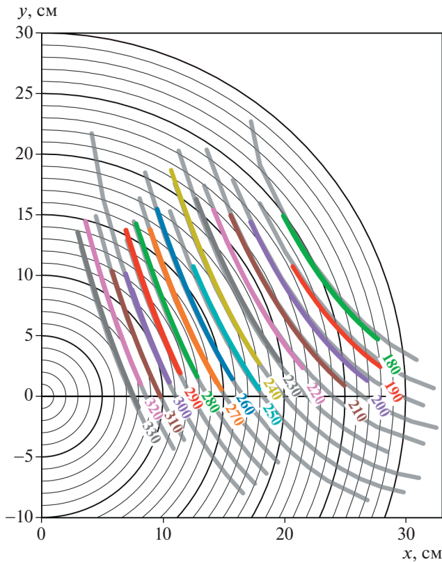
Рис. 5. Область измерения ЗПТИ для режима Т-10 с магнитным полем на оси B_z = 2.2 Тл, током плазмы I_{pl} = 230 кА. Цветные линии — детекторные линии равной энергии зондирующего пучка, полученные в результате измерений; серые — расчетная детекторная сетка. Энергия пучка E_{beam} = 180\text{--}330 кэВ.
