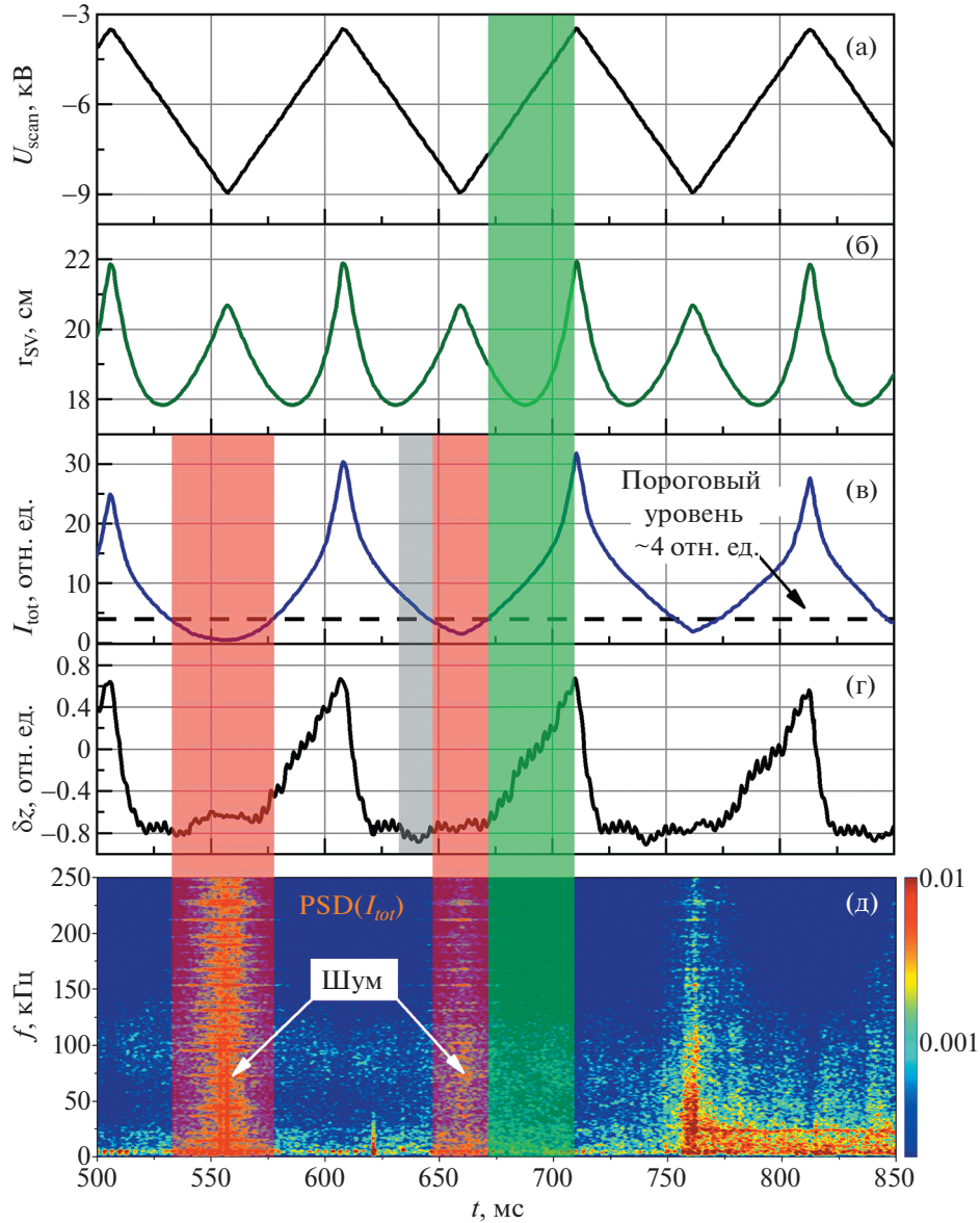
Рис. 6. Порядок разбиения сигналов ЗПТИ на отдельные сканы на примере импульса #73143 ( B_z = 2.2 Тл, I_{pl} = 230 кА, \bar{n}_e = 1.1 \cdot 10^{19} \text{ м}^{-3} , E_{beam} = 240 кэВ): а) напряжение на отклоняющих пластинах; б) временная эволюция радиального положения точки измерения r_{SV} ; в) полный ток с пластин детектора I_{tot} ; г) тороидальное смещение пучка на детекторе \delta z ; д) спектральная плотность мощности колебаний полного тока с пластин детектора; красным отмечены временные интервалы с высоким уровнем шума, непригодные для обработки; зеленым — временной интервал одного обрабатываемого скана; серым — интервал с превышением предельного значения \delta z .
